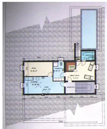
SUTERÉN
