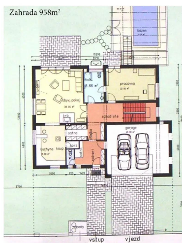
PŘÍZEMÍ
